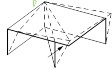
Labiles Verhalten sich kreuzender Scheiben unter Horizontallast
